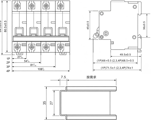
TH35-7.5型安装导轨尺寸
